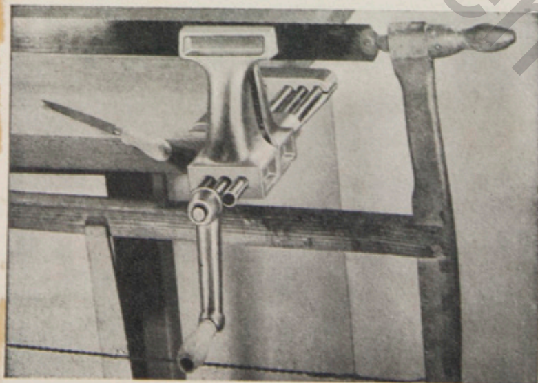
Les scies de toute nature y compris les scies de bûcheron, peuvent être fixées de cette façon dans les mâchoires.
