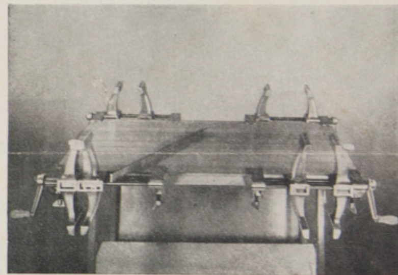
Que l'on soit droitier ou gaucher, peu importe où se trouve l'établi, ZYLYSS-HOBBY se pose aisément partout, exigeant une place minime.
