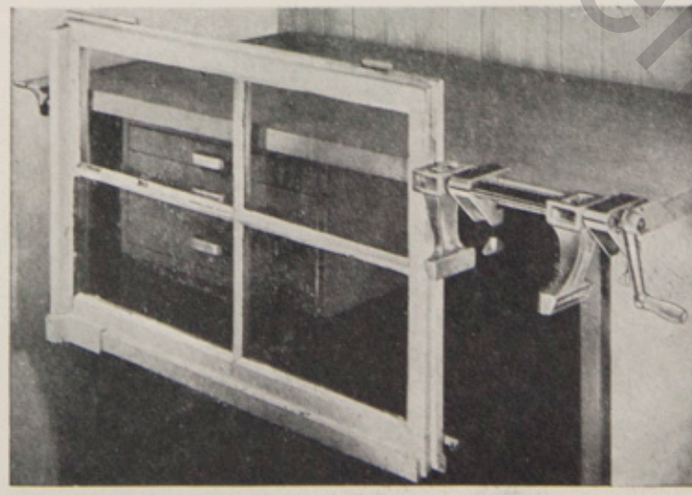
La retouche au rabot des feuillures de fenêtre ou de porte n'est plus un casse-tête avec ZYLYSS-HOBBY.
