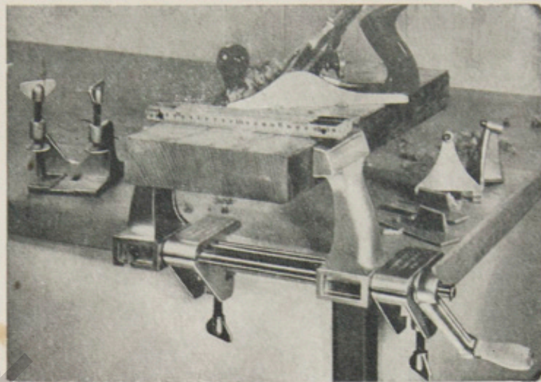
Cale N° 2 à l'intérieur des mâchoires = ZYLYSS-HOBBY permet même de fixer en toute sécurité de grosses pièces mesurant plus de 20 cm.
