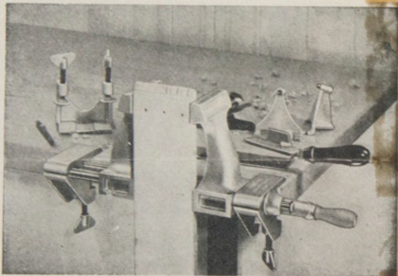
Même fixée verticalement, la pièce est toujours doublement tenue par les mâchoires parallèles.
