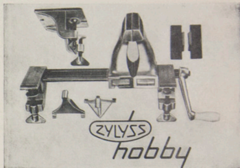
Pièces en fonte de métal léger trempé, guide mâchoires et écrous en acier poli; vis en acier comprimé, mâchoires en plastique incassable.
