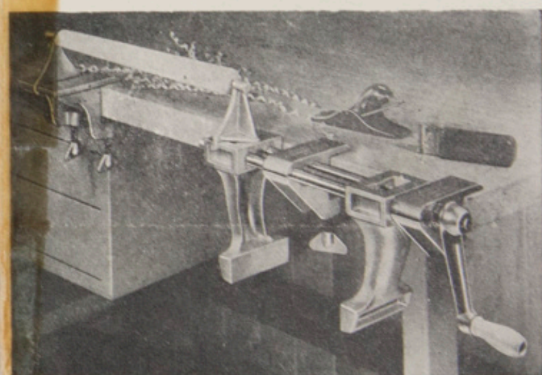
Serre-joint auxiliaire et mâchoires à tourner pour travailler les pièces polygonales ou rondes de toutes dimensions.
