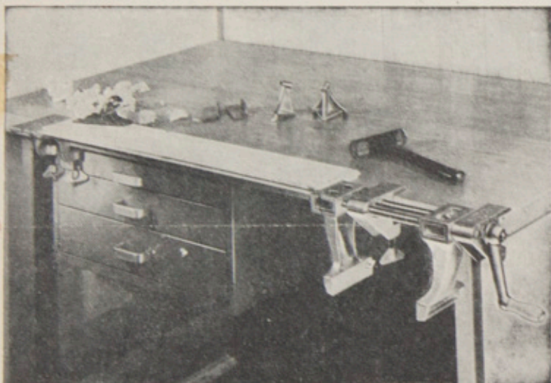
Cale N° 2 placée entre les mâchoires = l'utilisation du serre-joint auxiliaire permet de fixer des planches étroites de n'importe quelle longueur.
