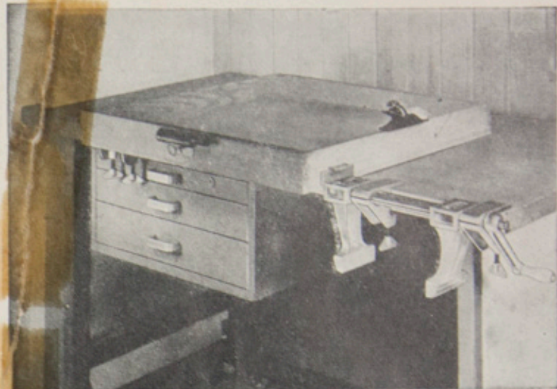
Les tiroirs ainsi que les pièces encombrantes se laissent aisément travailler de cette façon.
