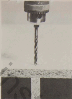
Perçer Ø 6 mm profondeur 62 mm
