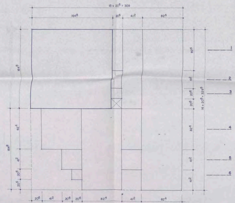
MODULO A ESC. 1:20
