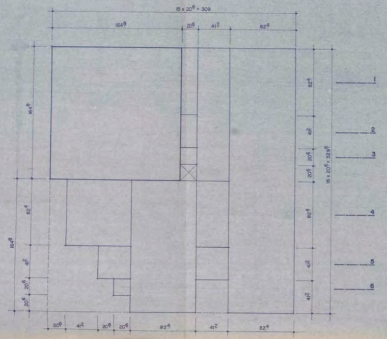
MODULO A ESC. 1:20
