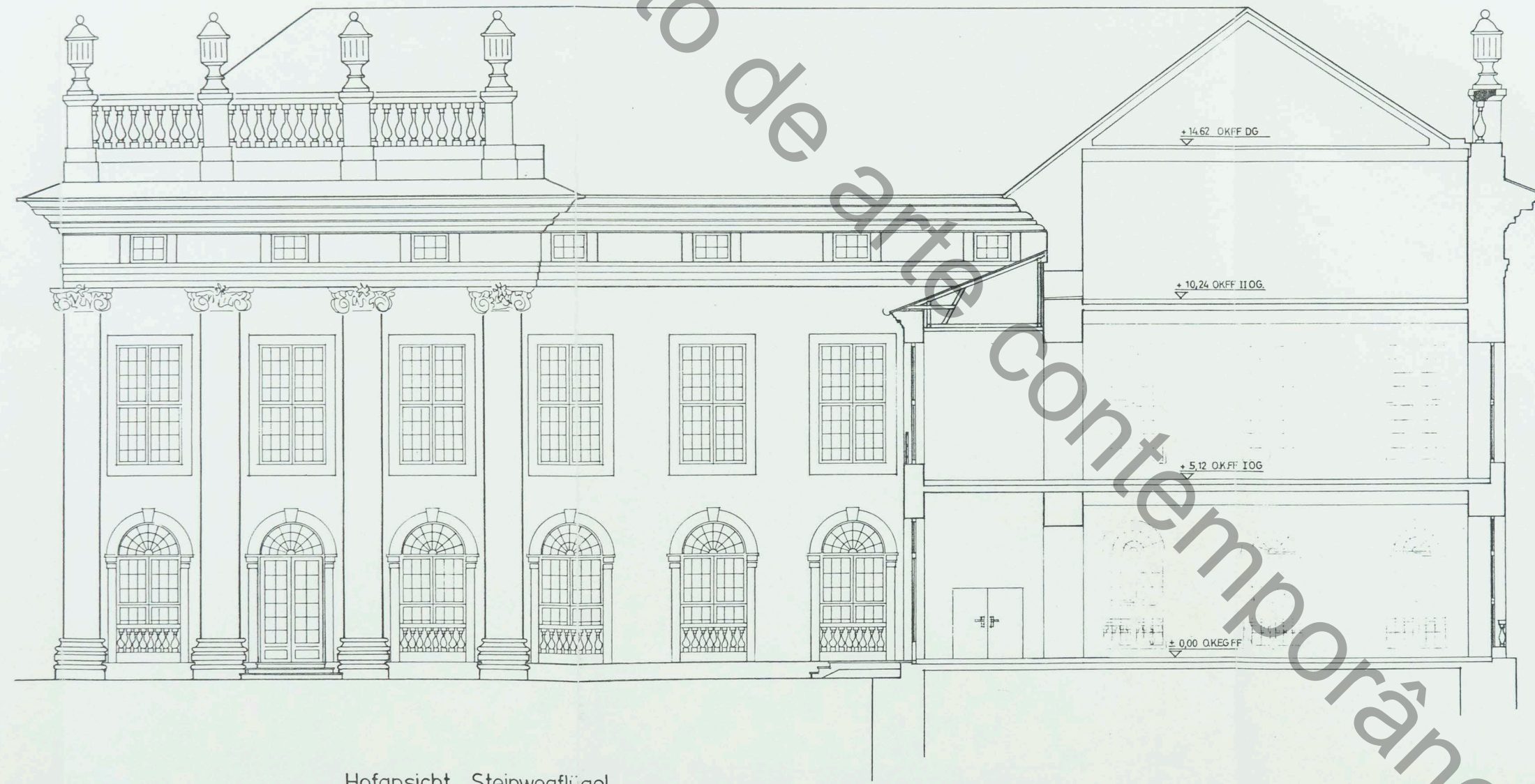
Hofansicht Steinwegflügel
